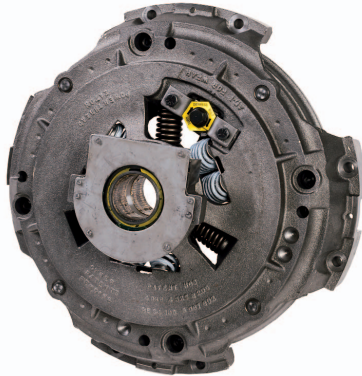
Easy-Pedal™ 2000 Clutch
